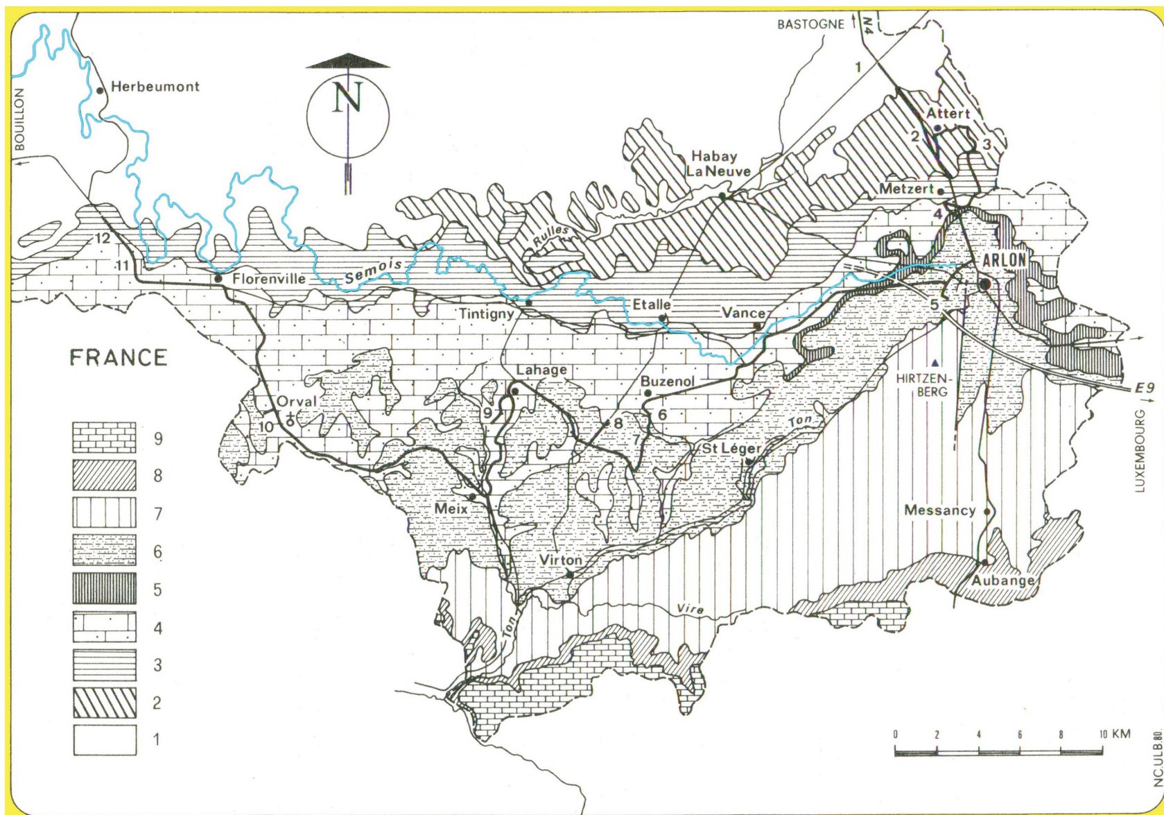
Carte géologique simplifiée du Sud-Luxembourg et itinéraire à travers le Trias et le Lias inférieur (extraite du guide géologique Belgique chez MASSON - 1983)
